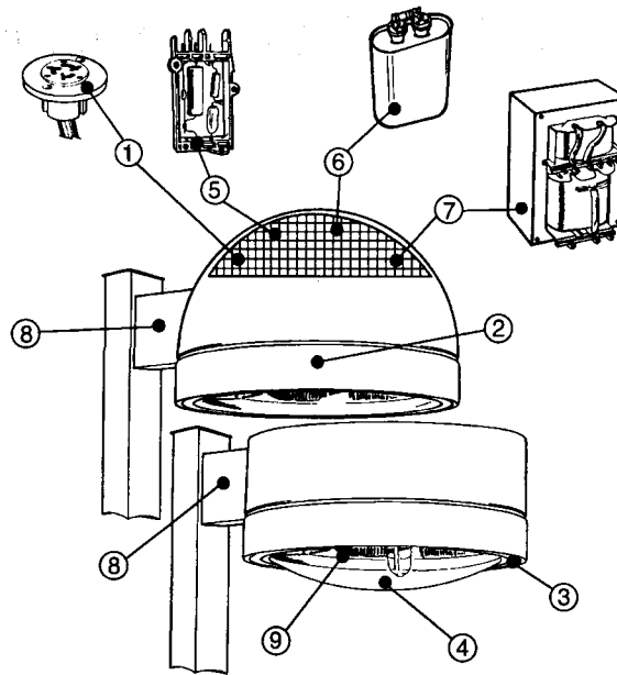
DECASPHERE™ LUMINAIRE
